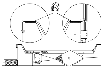
Einbau WESKO Duschwannenträger
