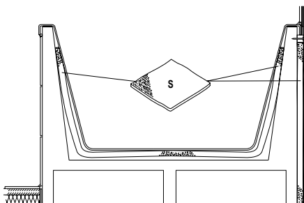
Einbau WESKO Badewannenträger E: WESKO Schallentkopplungsstreifen S: WESKO Schalldämpfungsmatten
